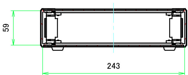
B-B ( 1:4 )
